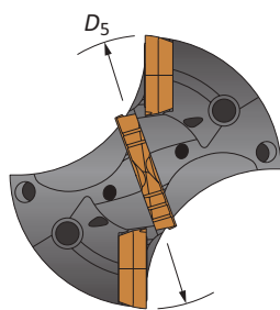
T-A® Head
