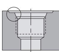
SAE J-1926-1 / ISO 11926-1
